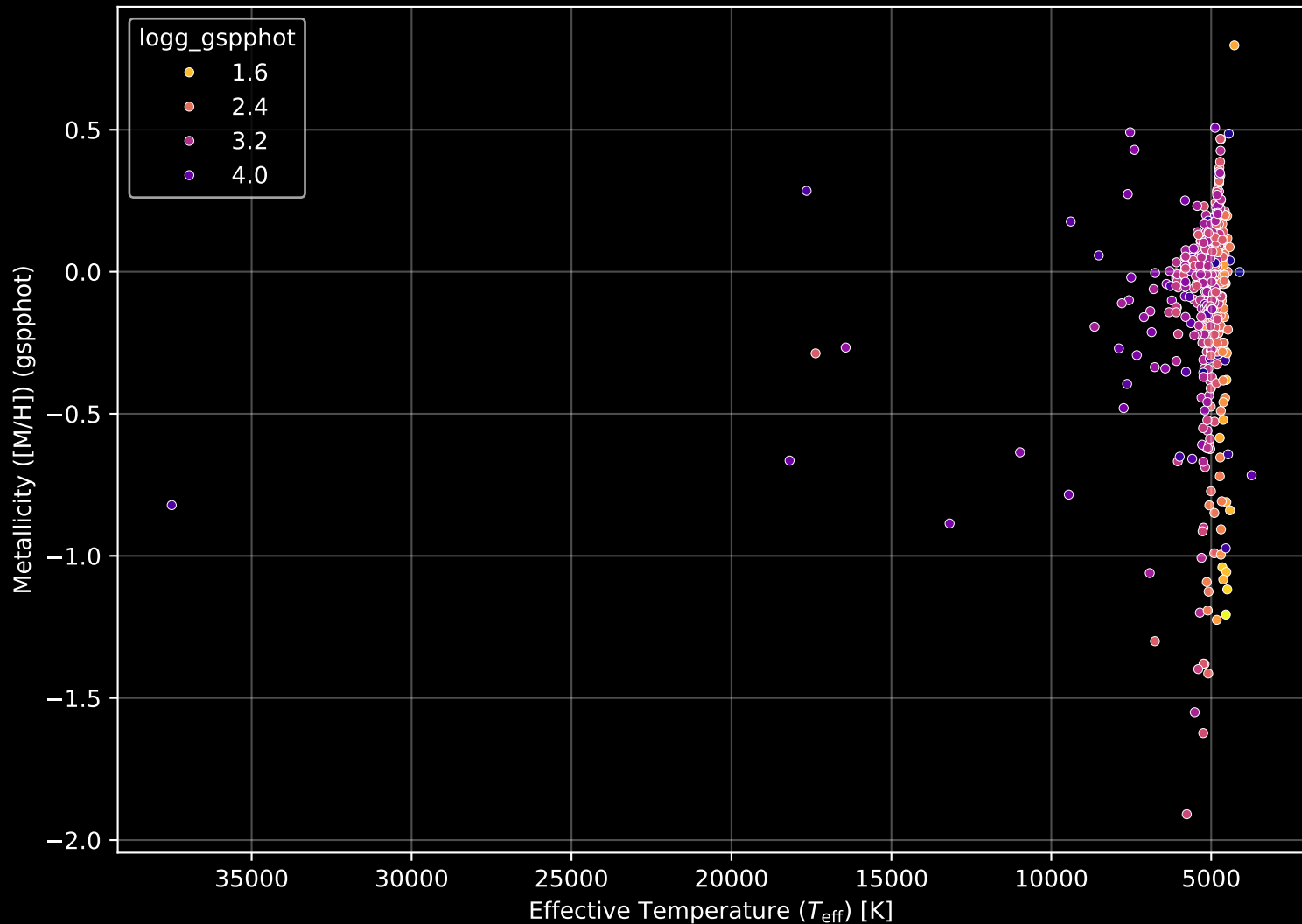
APOGEE DR17 Field: [100+06] Stellar Population Parameters (n= 556)
